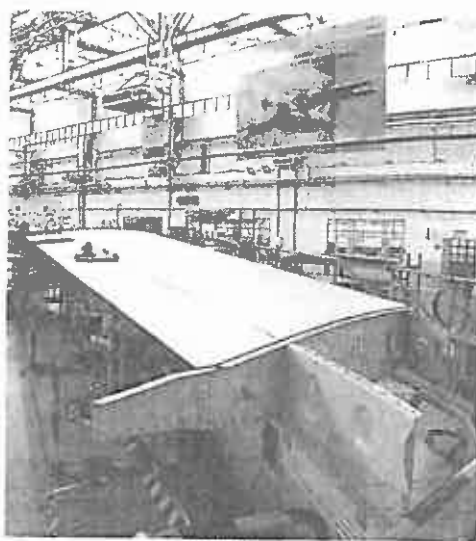
Uno de los cajones del estabilizador horizontal del A400M.
