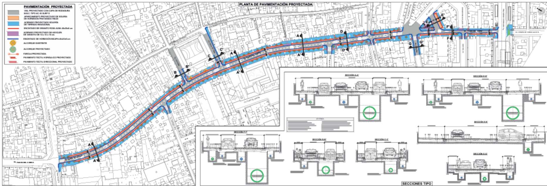
PLANTA DE PAVIMENTACIÓN PROYECTADA
